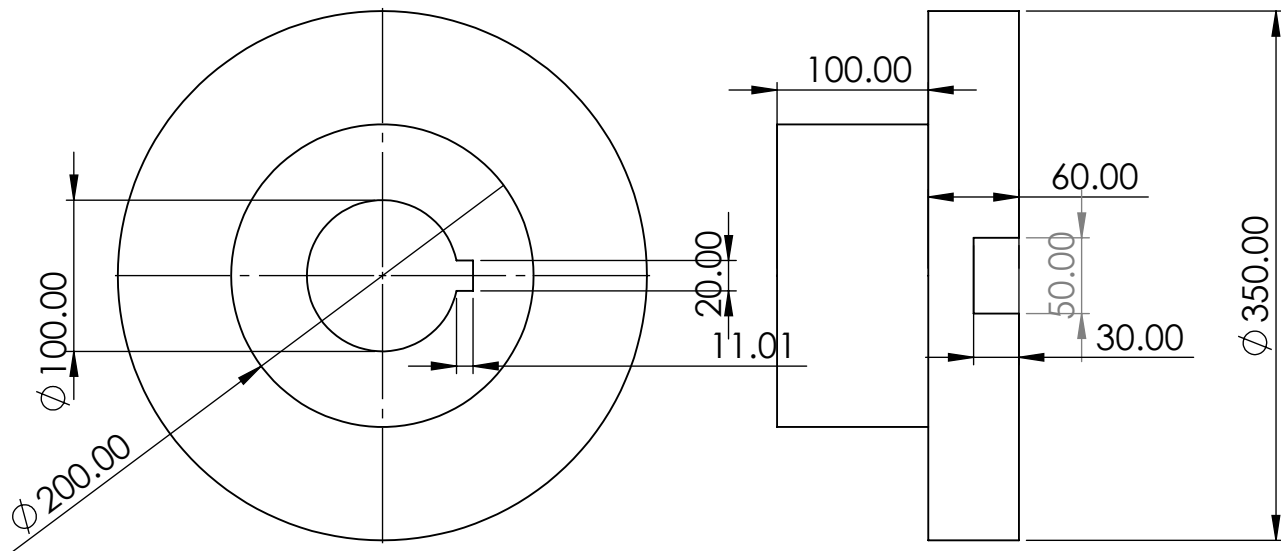
Flange
