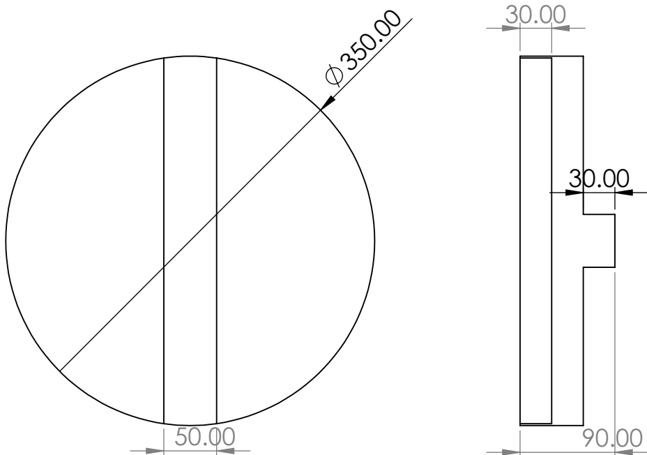
Flange
